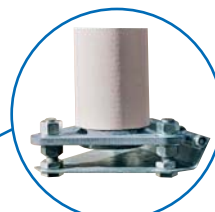
Platine basculante
